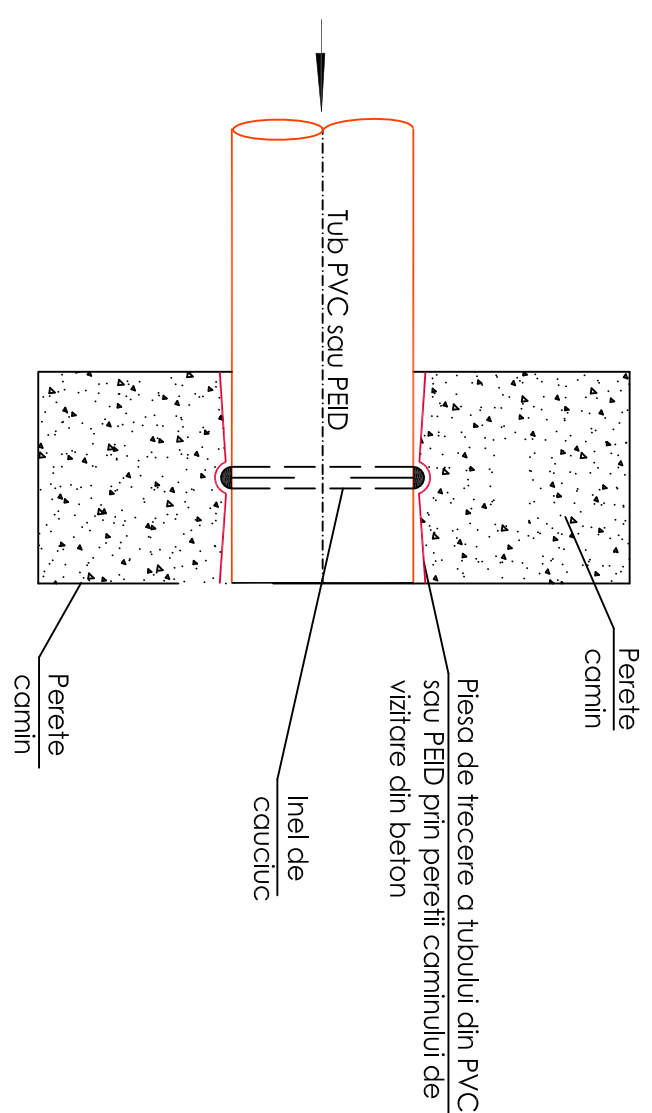
DETALIU "A" PIESA DE RACORDARE A TUBULUI DE PVC SAU PEID LA CAMINUL DIN BETON
