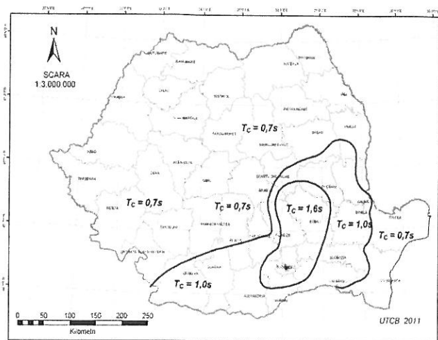
Fig 5. Zonarea teritoriului Romaniei in termeni de perioada de control (colt), T_c a spectrului de raspuns
