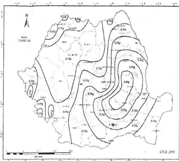
Fig 4.- Zonarea valorilor de varf ale acceleratiei terenului pentru proiectare ag cu IMR = 225 ani si 20% probabilitate de depasire in 50 de ani, conform P 100/1/2013
