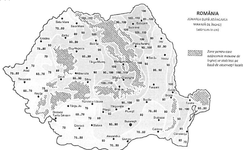
Figura 1. Zonarea adancimii de inghet, conform STAS 6054/77
